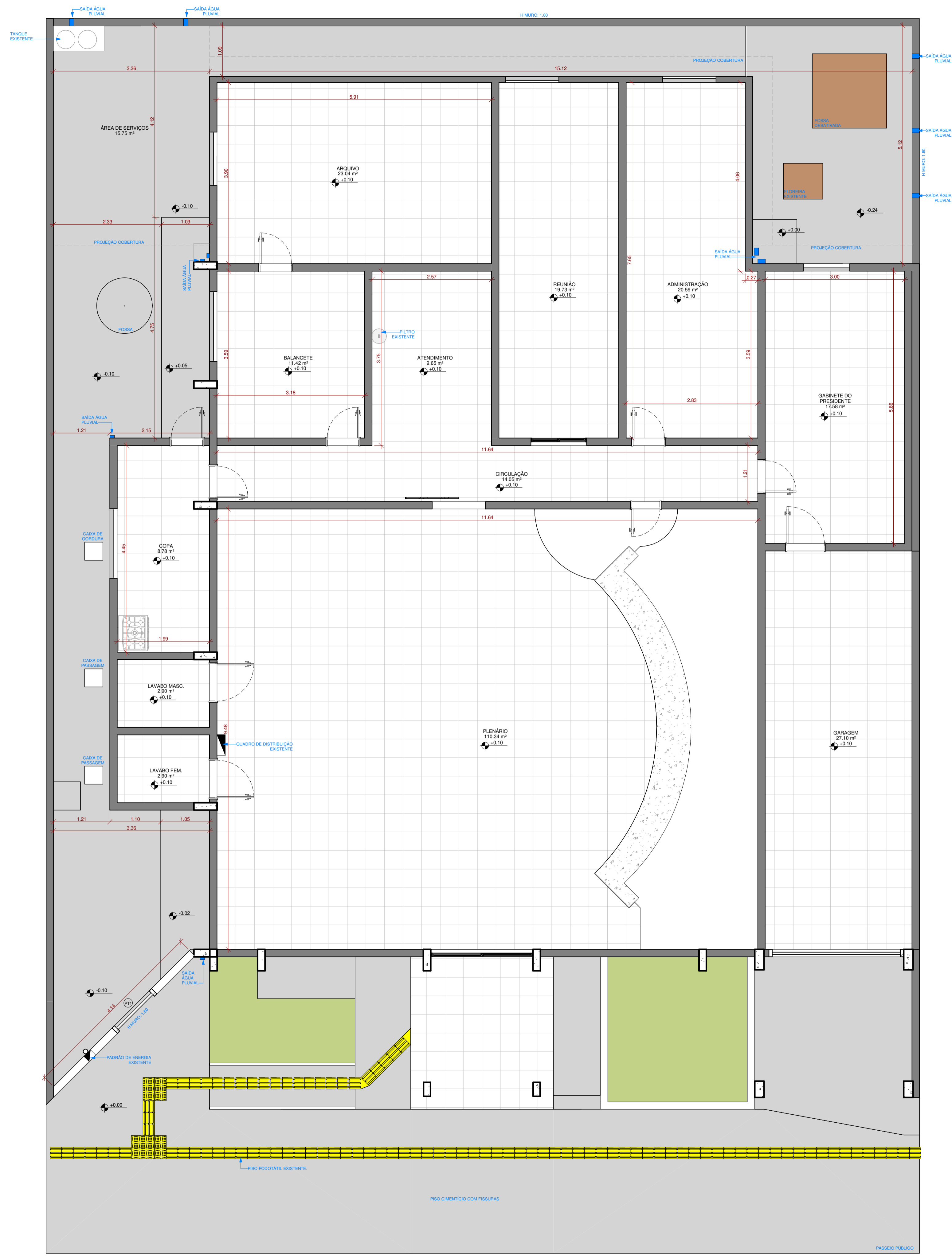
01 PLANTA BAIXA TÉRREO - LEVANTAMENTO ESCALA 1:50
