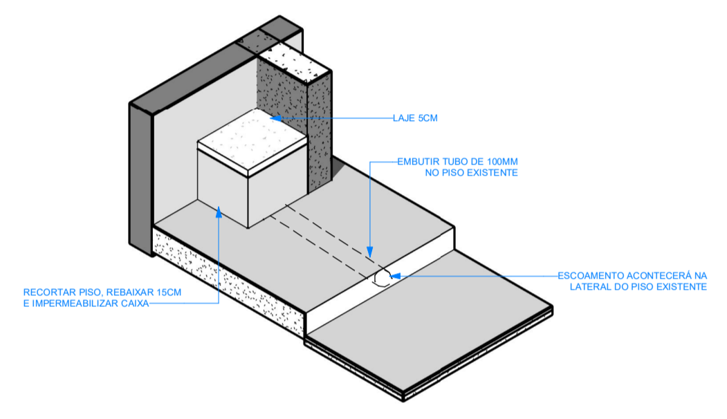
02 DET. CX PASSAGEM ESCALA
