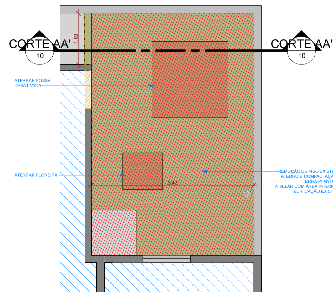
04 PLANTA MOVIMENTAÇÃO DE TERRA ESCALA 1:50
