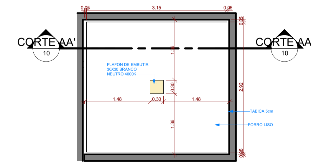
08 PLANTA DE FORRO ANEXO 02 - SALA ESCALA 1:50
