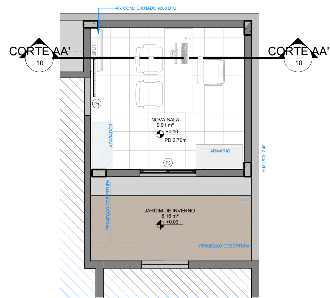
01 PLANTA DE LAYOUT ANEXO 02 - SALA ESCALA 1:50
