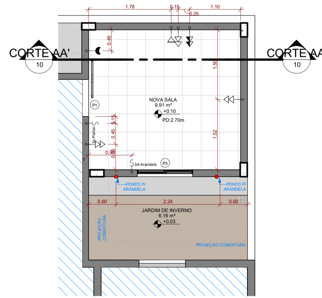
06 PONTOS ELÉTRICOS ANEXO 02 - SALA ESCALA 1:50
