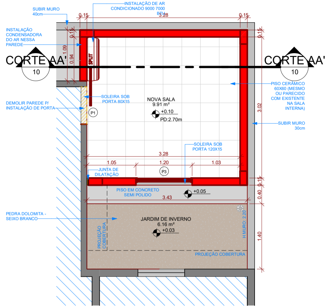
02 PLANTA DE REFORMA ANEXO 02 - SALA ESCALA 1:50
