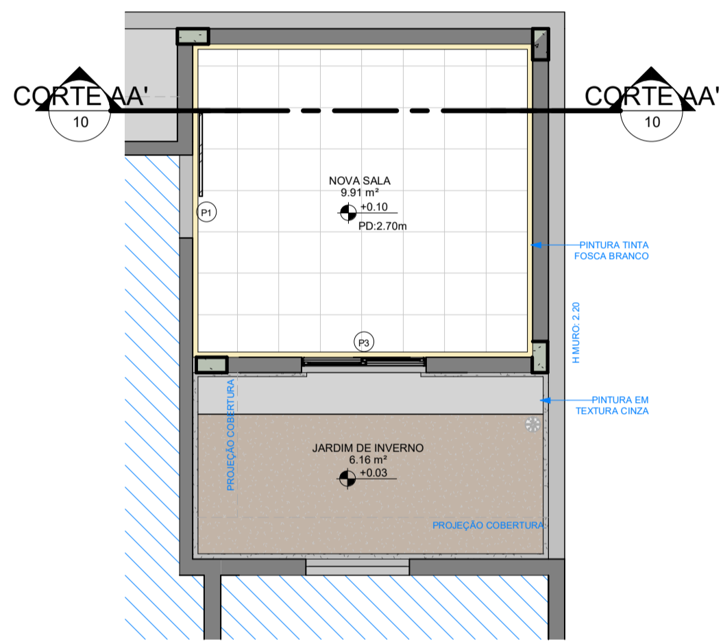
05 PLANTA DE REVESTIMENTOS ANEXO 02 - SALA ESCALA 1:50
