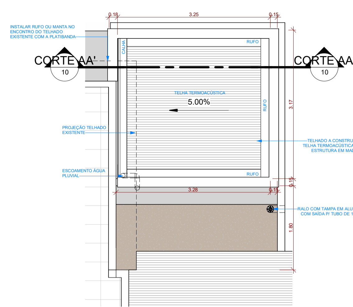
03 PLANTA DE COBERTURA ANEXO 02 - SALA ESCALA 1:50
