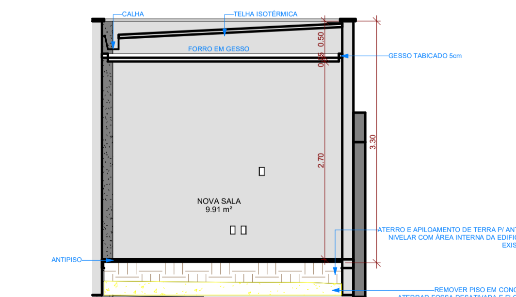
07 CORTE AA' ESCALA 1:50
